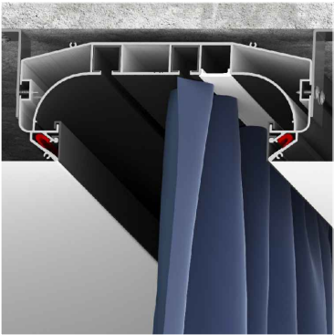
Профиль LumFer SK Magnum
